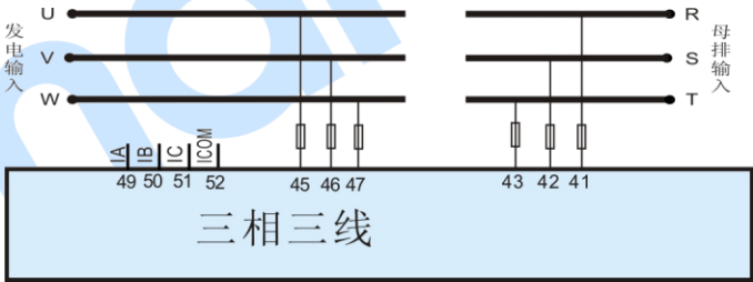
图5 三相三线应用图
