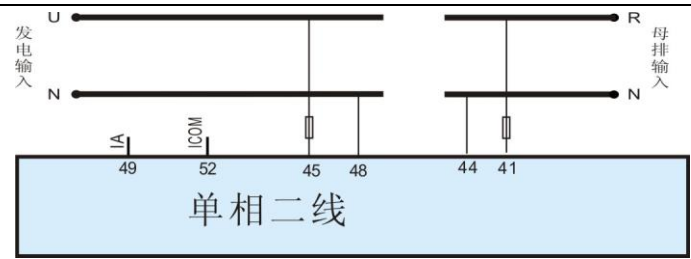
图7 单相二线应用图
