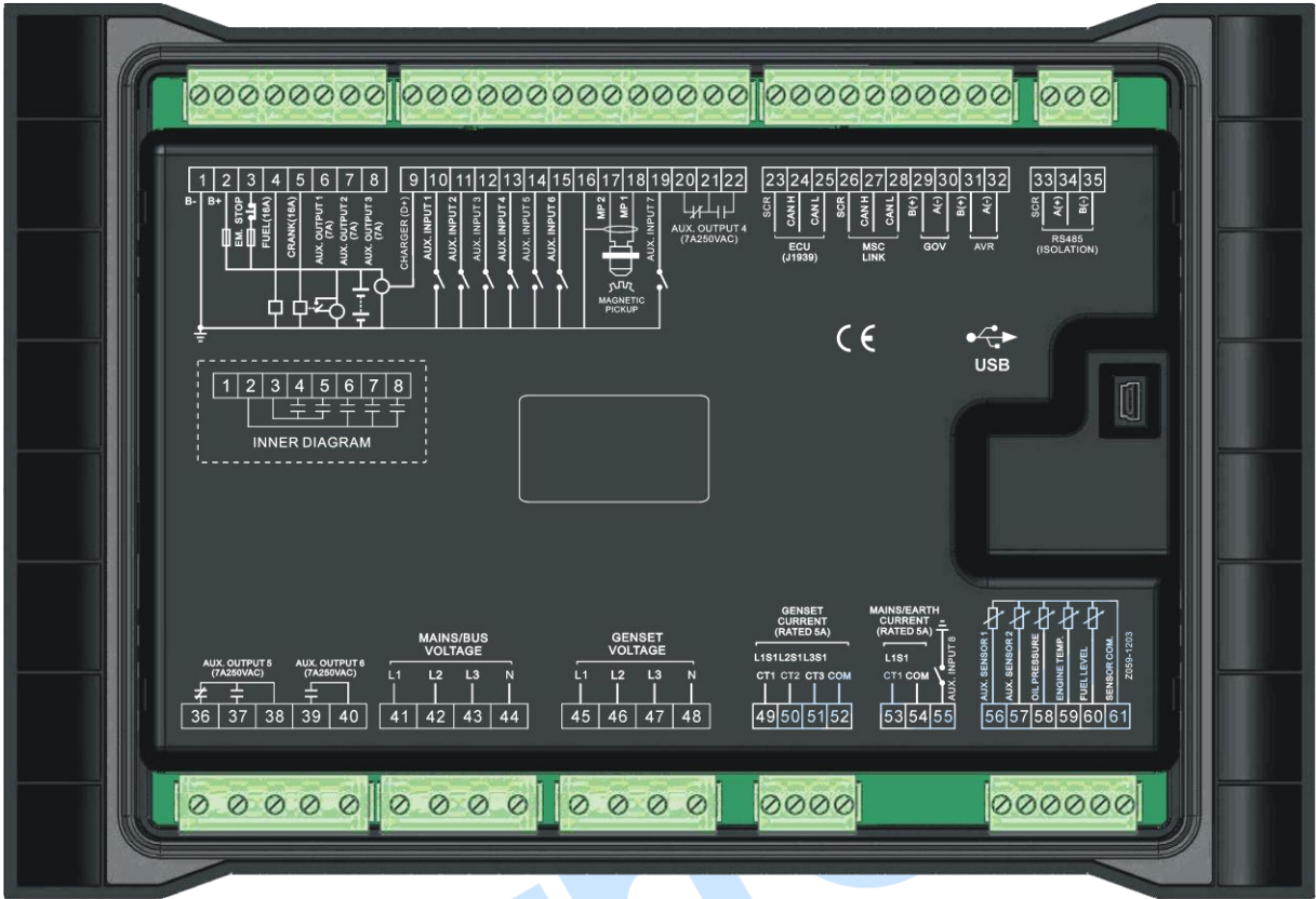
图2 HGM9510 控制器背面板
