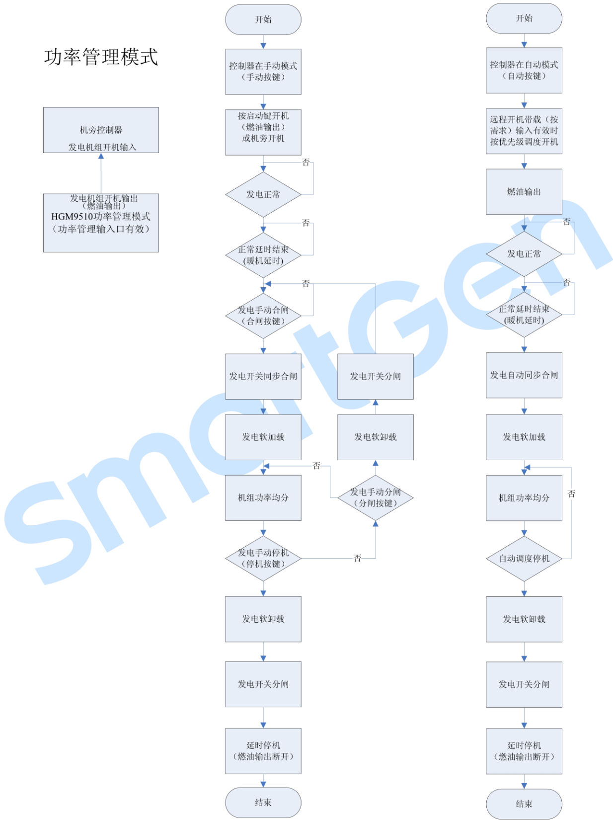
图9 功率管理逻辑
