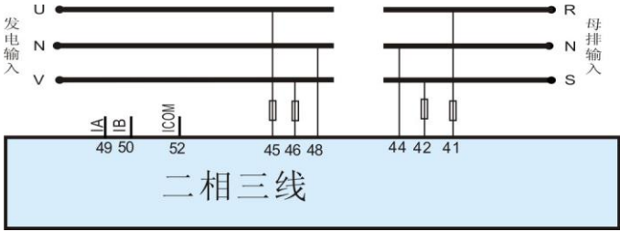
图6 二相三线应用图
