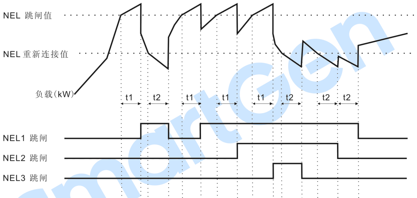
图10 NEL 时序
