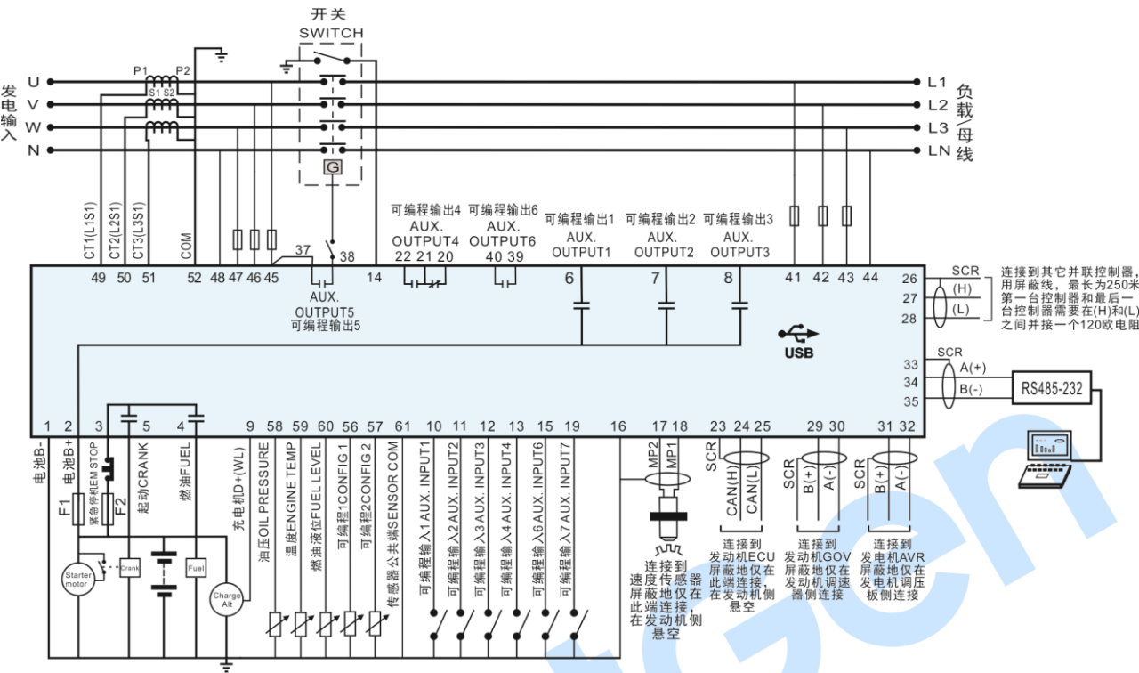
图4 HGM9510 三相四线典型应用图
