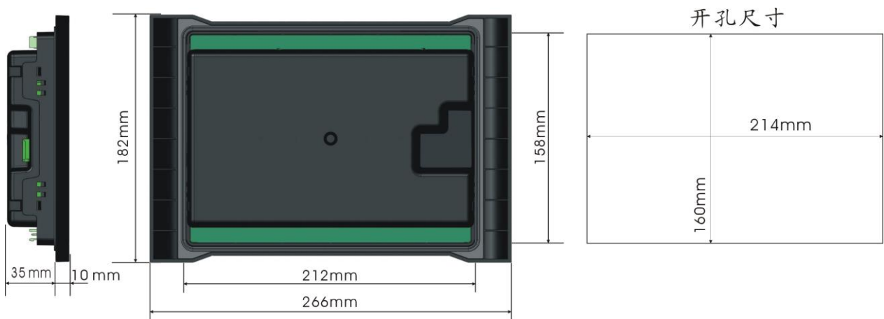
图11 外形尺寸及面板开孔尺寸
